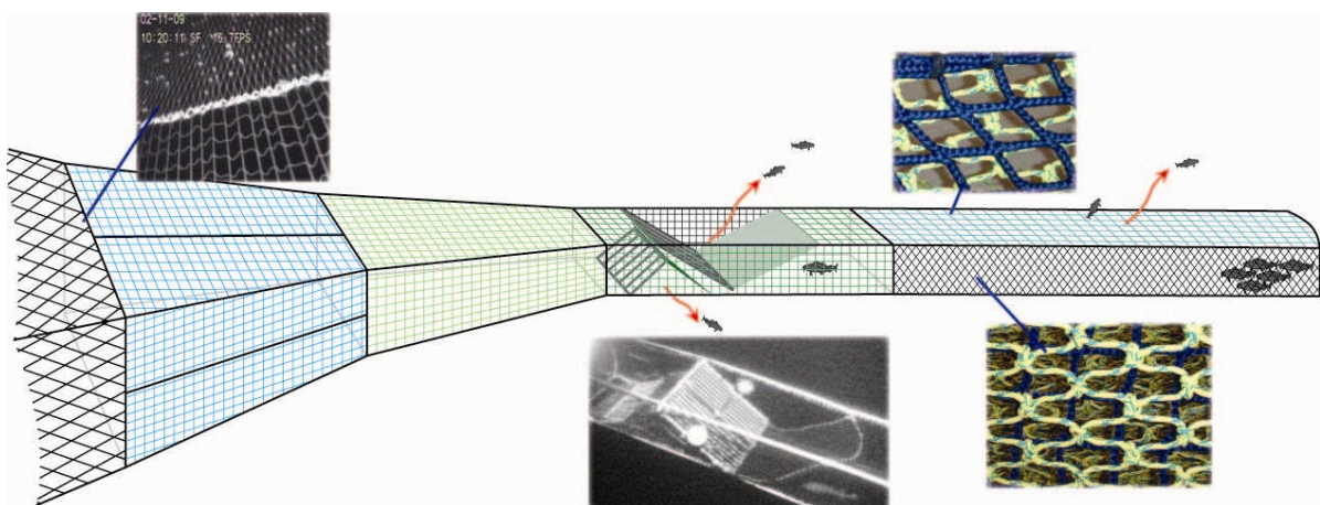
Bilde 2. Det nye konseptet for konstruksjon av bakparten av flytetrålen. Belg/forlengelse i kvadratmaskepanel, rist i 4-panels seksjon i kvadratmasker og pose med kvadratmasker i overpanel og T90 masker i side og underpanel.
